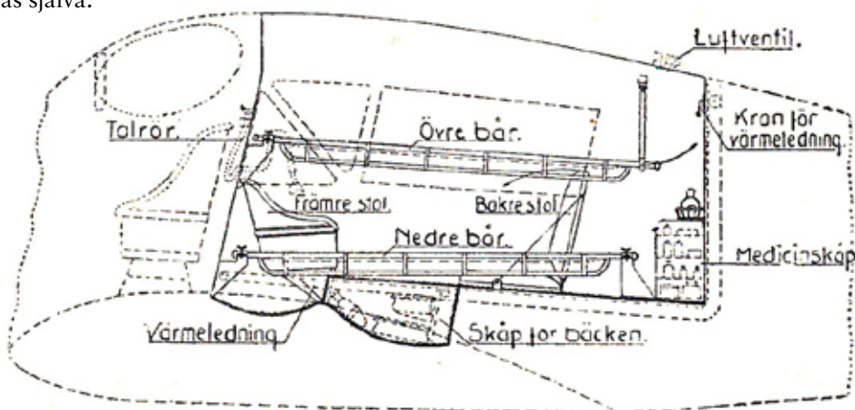
I tidningen Levande livet från 1934 publicerades en ritning över en dåtida modern sjukhytt på ett flygplan. Sjukhytten har två båar och ett talrör mellan kabinen och cock-pit.
